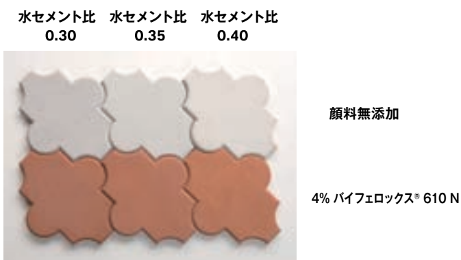
図2：水セメント比とコンクリートの発色の関係
